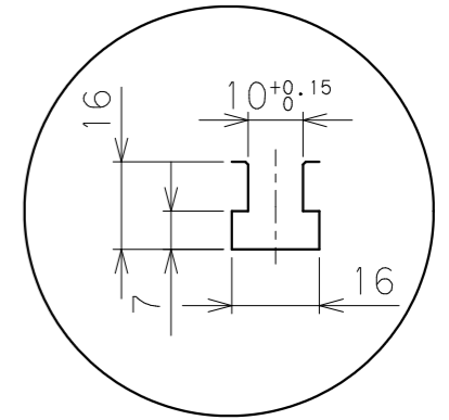
A部詳細2 : 1
