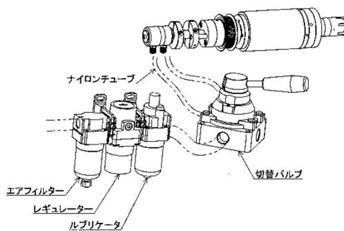
空気圧補助機器類取付け例
