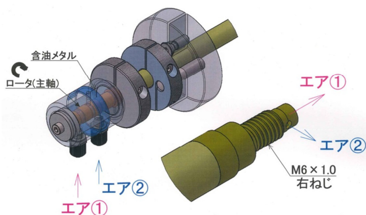
図 2 P 部、Q 部詳細図
