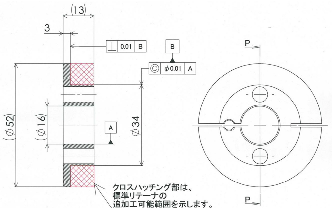
断面图 P-P
