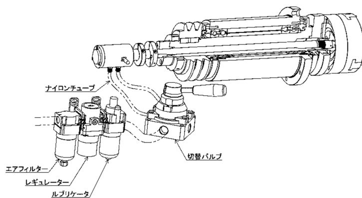
空気圧補助機器類取付け例
