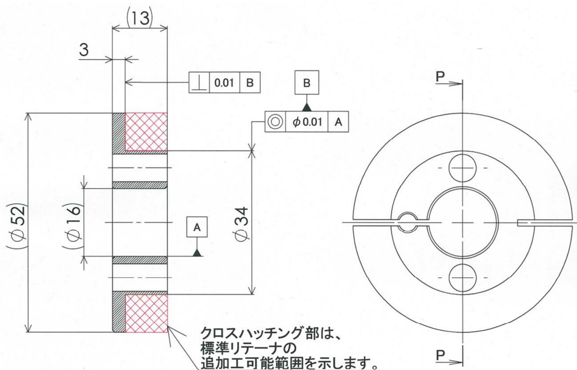
断面图 P-P
