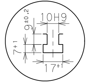
A部詳細2:1
