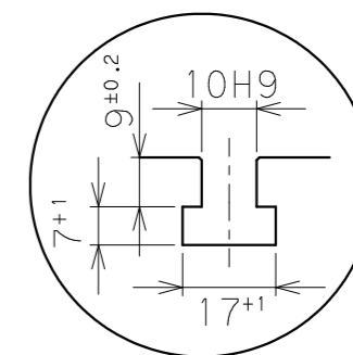
A部詳細2:1
