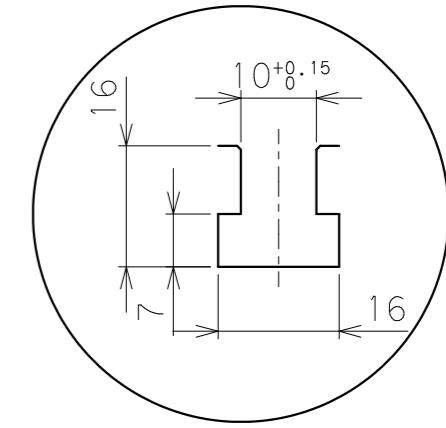
A部詳細2:1
