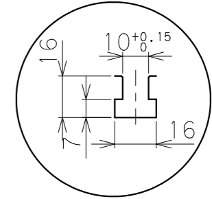
A部詳細2:1
