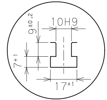
A部詳細2:1
